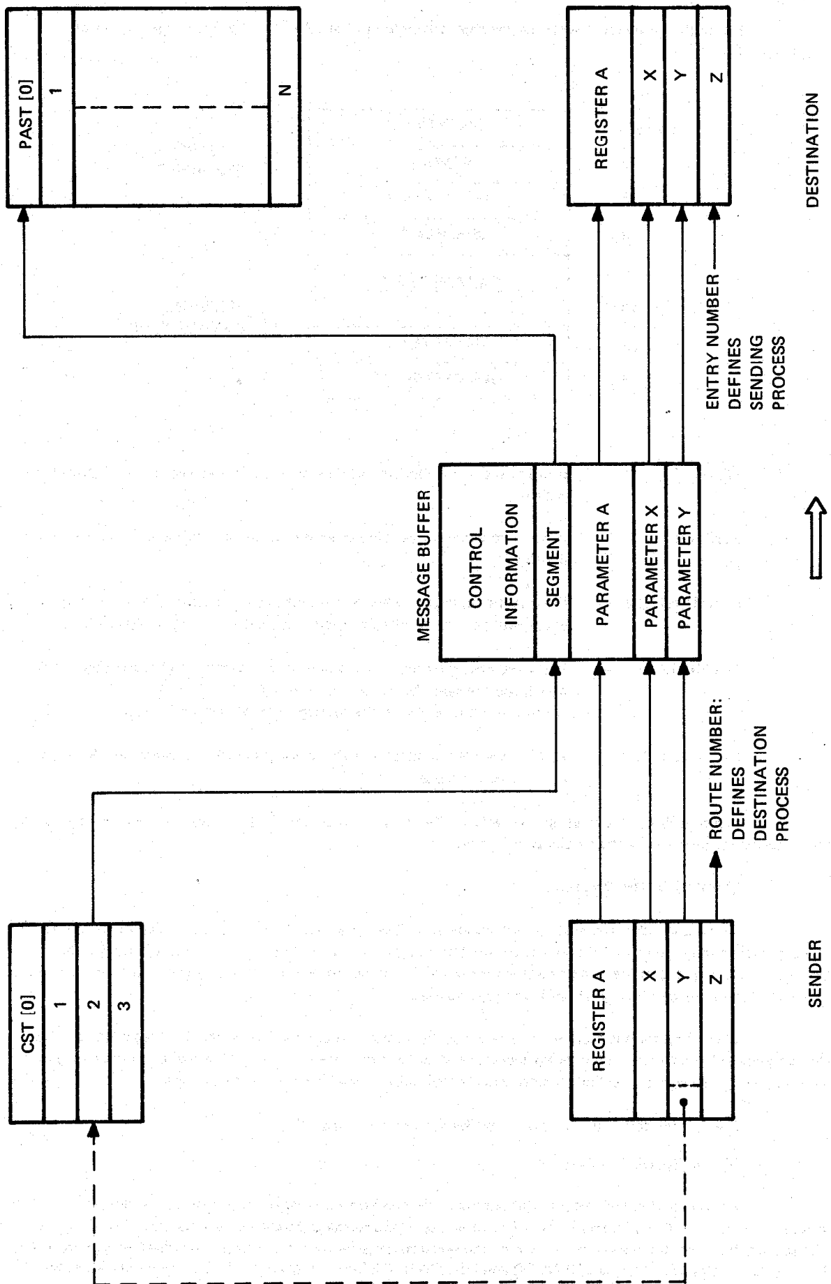
Figure 5: MESSAGE PARAMETERS
